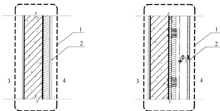
图 1 外围护结构外表面示意图
