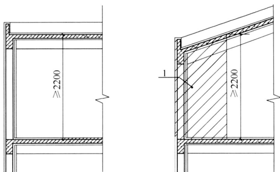
图2 结构层高或斜面结构板顶高度 在 2.20m 及以上的建筑空间示意图 1—不计算建筑面积的区域
