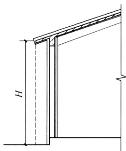
图 6 檐口高度计算示意图
