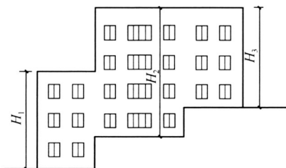
图 8 建筑高度计算示意图
