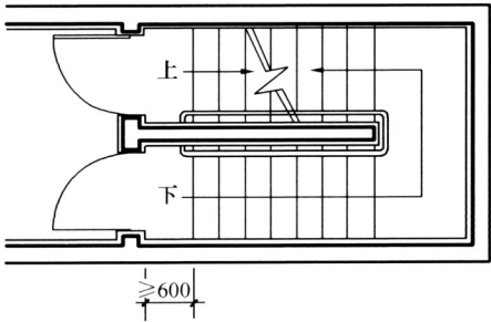
图 10 正对梯段设置的楼梯间门距踏步边缘的最小安全距离示意图
